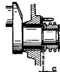
Fig. 3. REGLAGE DU LATERAL
