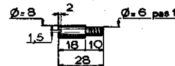
Fig. 4 - GOIJONS MR-3400 non vendus
