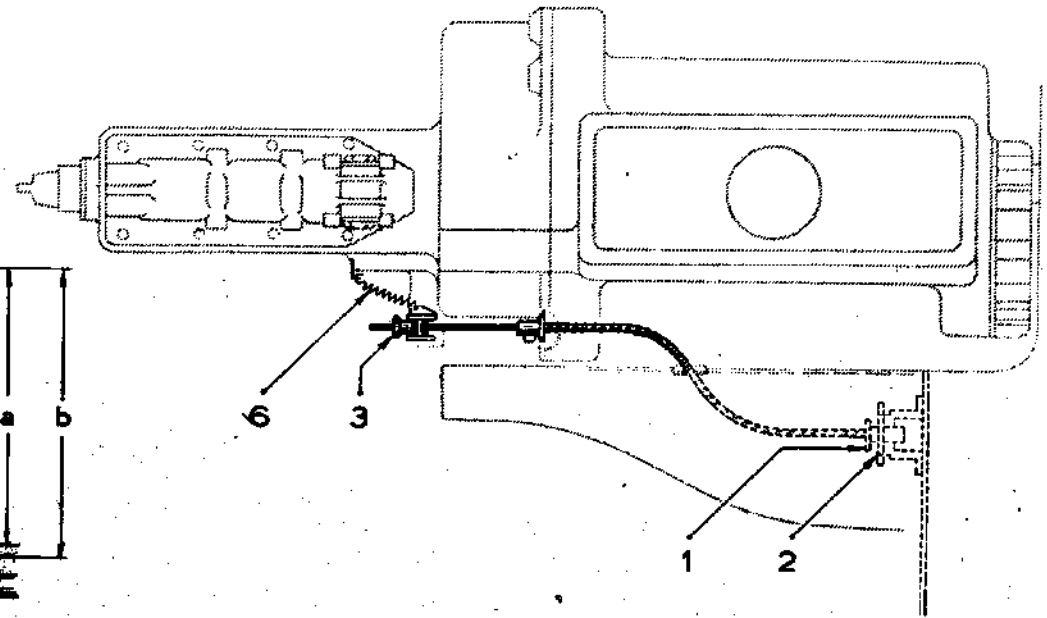
Fig 3 - MONTAGE DE LA GAINE
