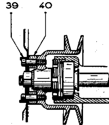
Fig. 4 - GOIJONS MR-3400 non vendus
