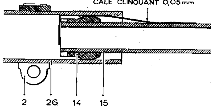
Fig. 3 CALE CLINQUANT 0,05 mm
