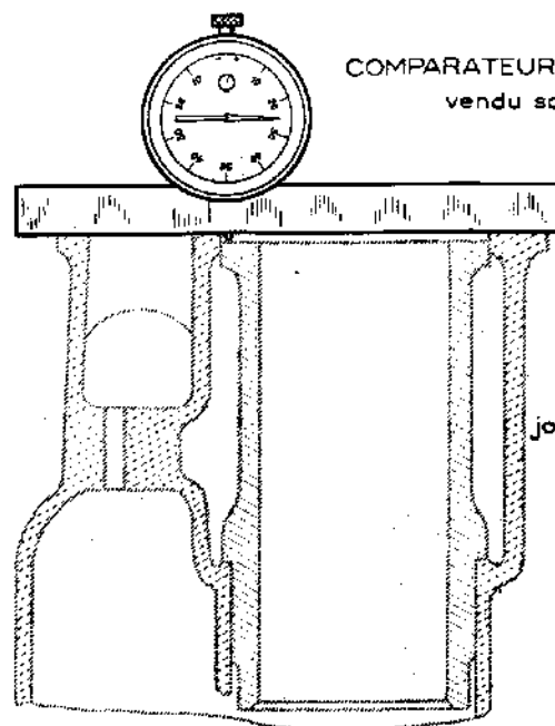
Fig. 3 - REGLE MR-3377 non vendue
