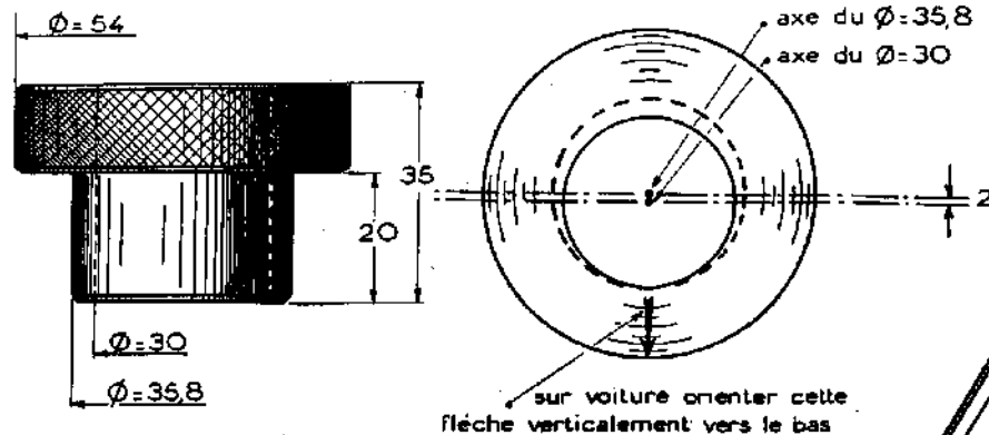
Fig. 3 _ FOURCHE vendue sous le n°1952-T
