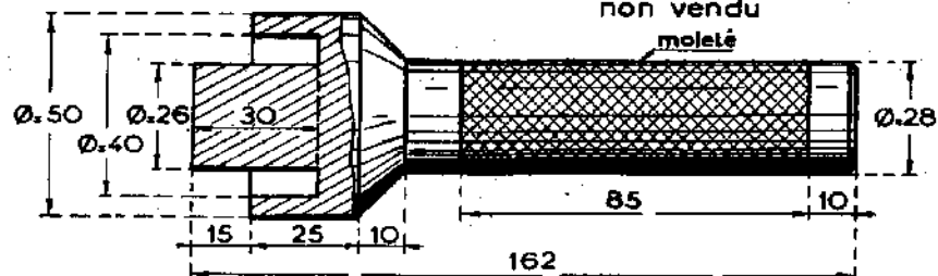
Fig 4 - MANDRIN MR-3602-10
