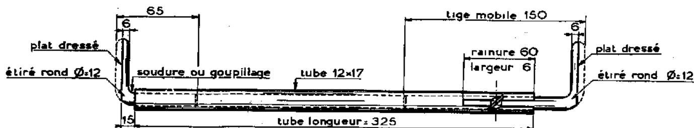
Fig. 2 - PIGE MR-3340-10 non vendue
