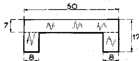
Fig. 3 - CALE MR-3505-20 non vendue
