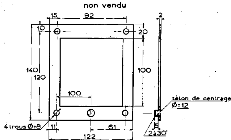
Fig. 4 - CALIBRE MR-4078-10
