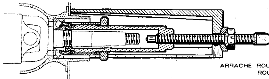
Fig. 3- EXTRACTION DU ROULEMENT INTERIEUR
