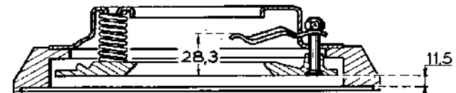
Fig 3 _ CONTROLE DU REGLAGE
