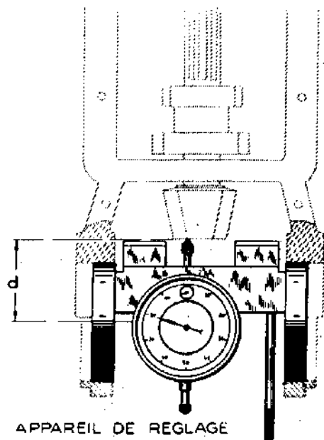
Fig 1 _ REGLAGE DE LA DISTANCE CONIQUE
