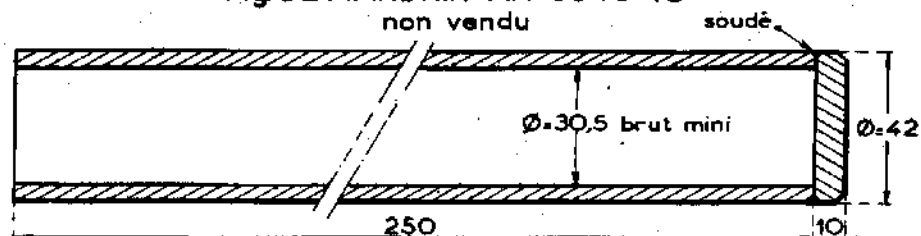
Fig 4 - MANDRIN MR-3602-10
