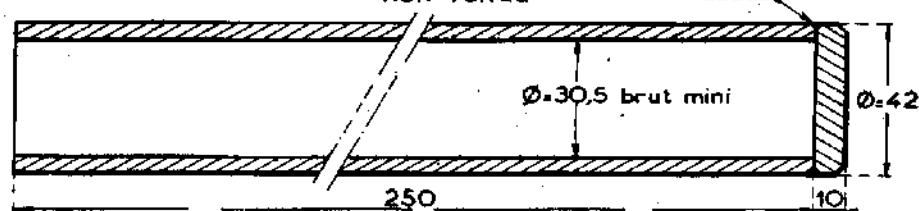
Fig 4 - MANDRIN MR-3602-10
