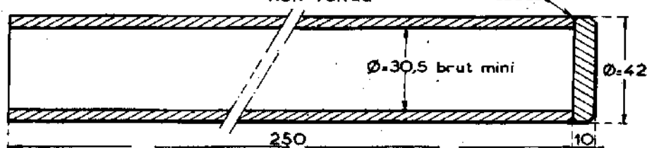
Fig 4 - MANDRIN MR-3602-10
