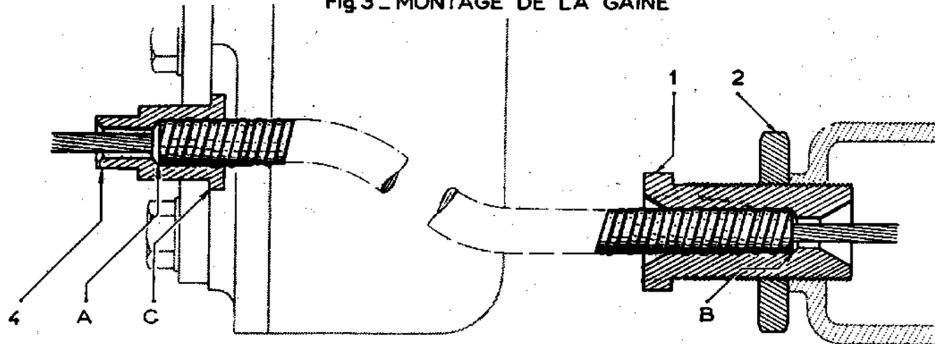
Fig 3 - MONTAGE DE LA GAINE
